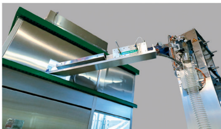
Ориентатор и стерилизация крышек/ Orientator and sterilization of the caps
